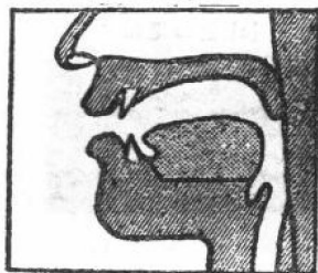
[u] 的口腔图
