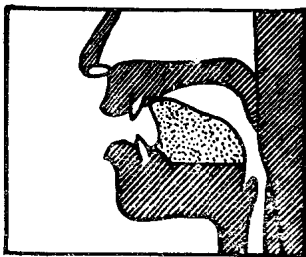
[t], [d] 的口腔图
