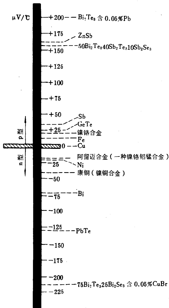
图 1.2 以铜为偶,在室温下测得的一些材料的塞贝克系数。
