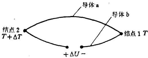
图 1.1 塞贝克效应的示意图
