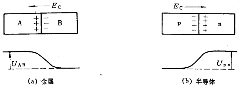
图 1.4 接触电动势的产生
