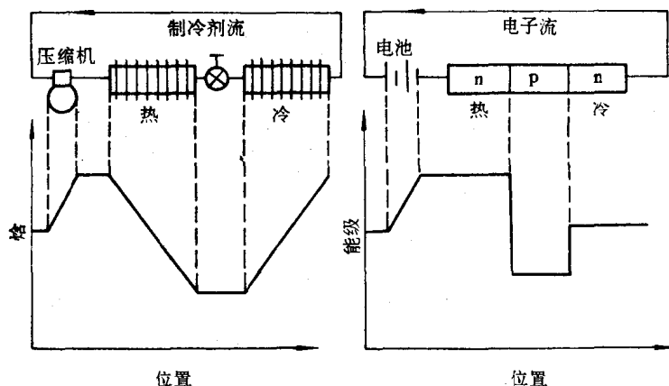
图 1.11 能级类似
