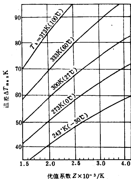
图 1.12 Z-\Delta T_{\max} 关系
