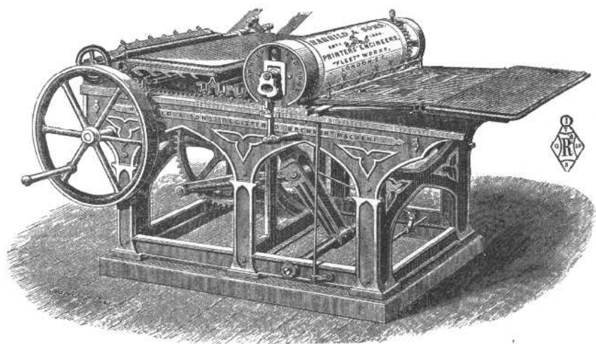
清同治十一年(1872年)申报馆从国外引进的手摇平台印刷机
