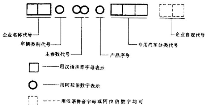
图 1-21 汽车产品型号构成
