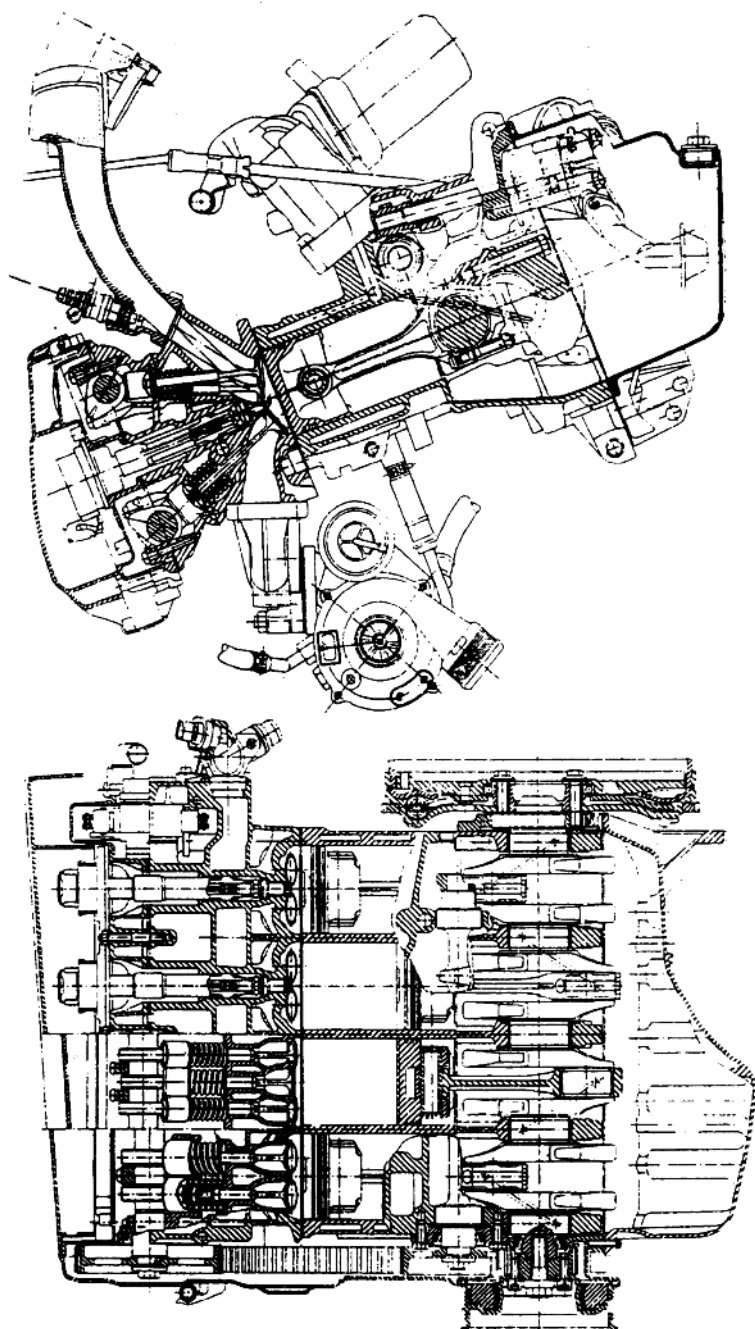
图 1-24 奥迪轿车发动机
