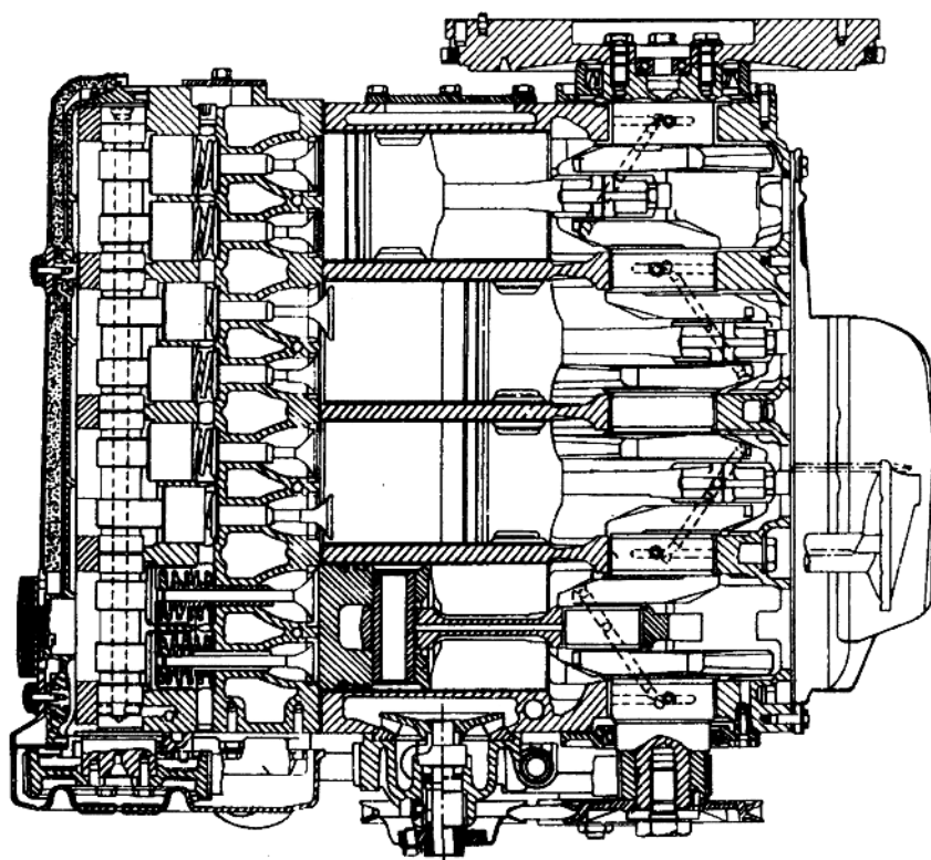
图 1-26 依维柯汽车用柴油机
