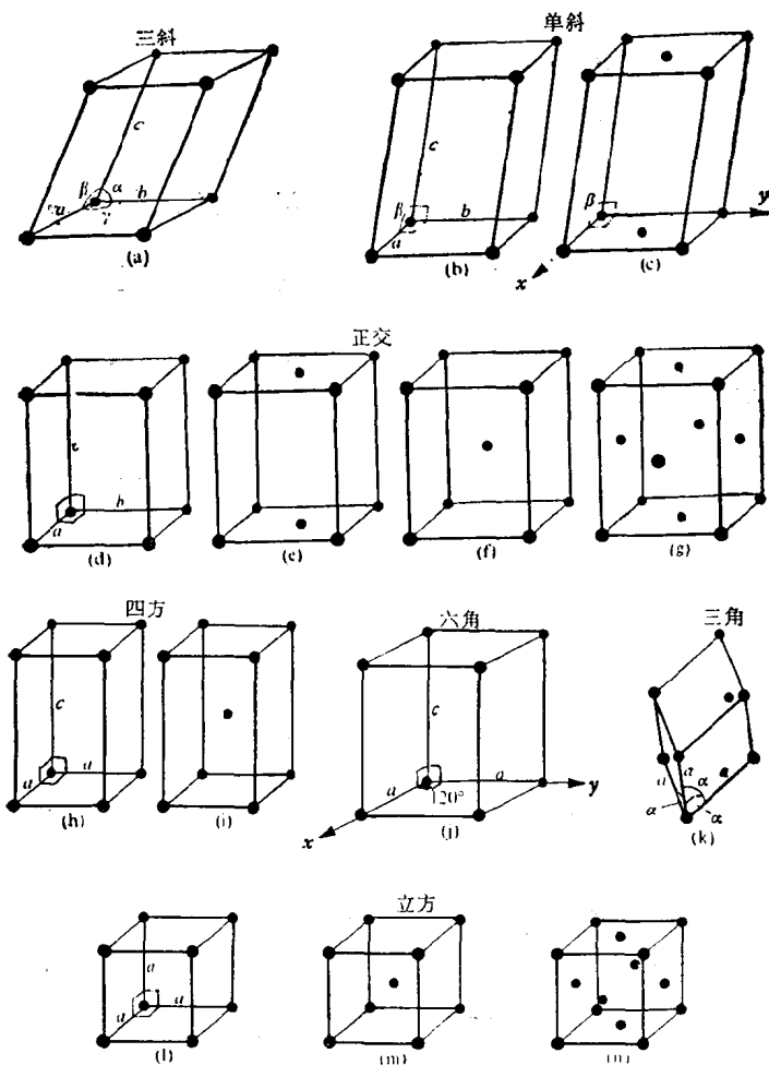
图1.1 14种布喇菲空间点阵的晶胞。(a) 简单三斜 (P); (b) 简单单斜 (P); (c) 底心单斜——通常取二次轴平行于 y 轴, 并取 (001) 为有中心的面 (C 中心); (d) 简单正交 P; (e) 底心正交——通常在 (001) 面上 (C 中心); (f) 体心正交 (I); (g) 面心正交 (F); (h) 四方 P; (i) 四方 I; (j) 六角 P; (k) 简单菱面体 (三角 R); (l) 立方 P; (m) 立方 I (体心立方); (n) 立方 F (面心立方)。
