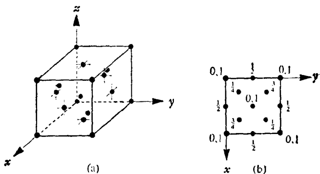
图1.3 金刚石结构的晶胞(a)和从 z 轴向下的投影(b)。这种结构具有面心立方点阵[见图1.1(n)]，每一阵点含有两个原子。
