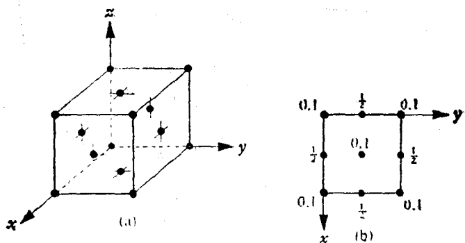
图1.2 面心立方结构的晶胞和投影。(a) 面心立方结构的晶胞[见图1.1(n)]。图中已标明结构位置的坐标。在这种结构中，通常假设原子是沿着立方体各个面的对角线方向( \langle 110 \rangle 方向)而保持接触的，称这种结构为密堆积结构；(b) 面心立方结构沿 z 轴向下的投影。在结构位置旁边的坐标以沿 z 轴的重复周期为单位。
