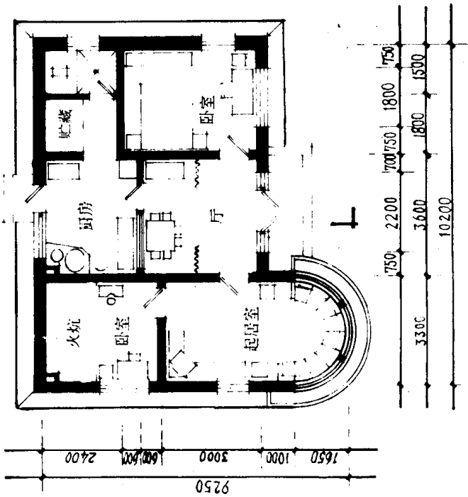
平面图
