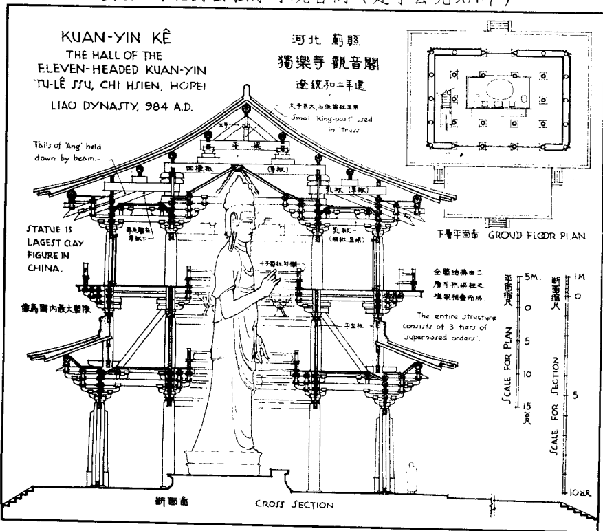
辽代建筑，河北蓟县独乐寺观音阁（建于公元984年）
