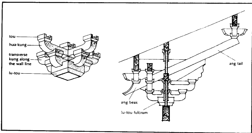
中国斗拱架，左图为复合架，右图为柱子上安放的斗拱架。
