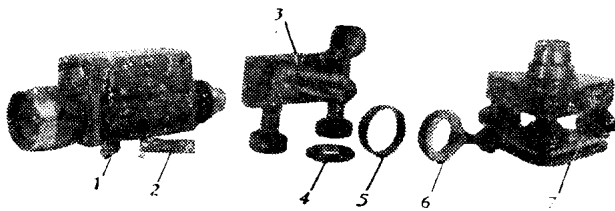
图12-5 照准部托板
