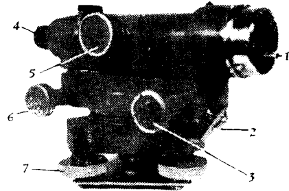
图13-1 CSZ030型水准仪外貌
