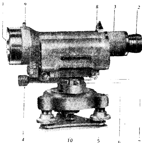
图14-1 ND 1 型水准仪外貌
