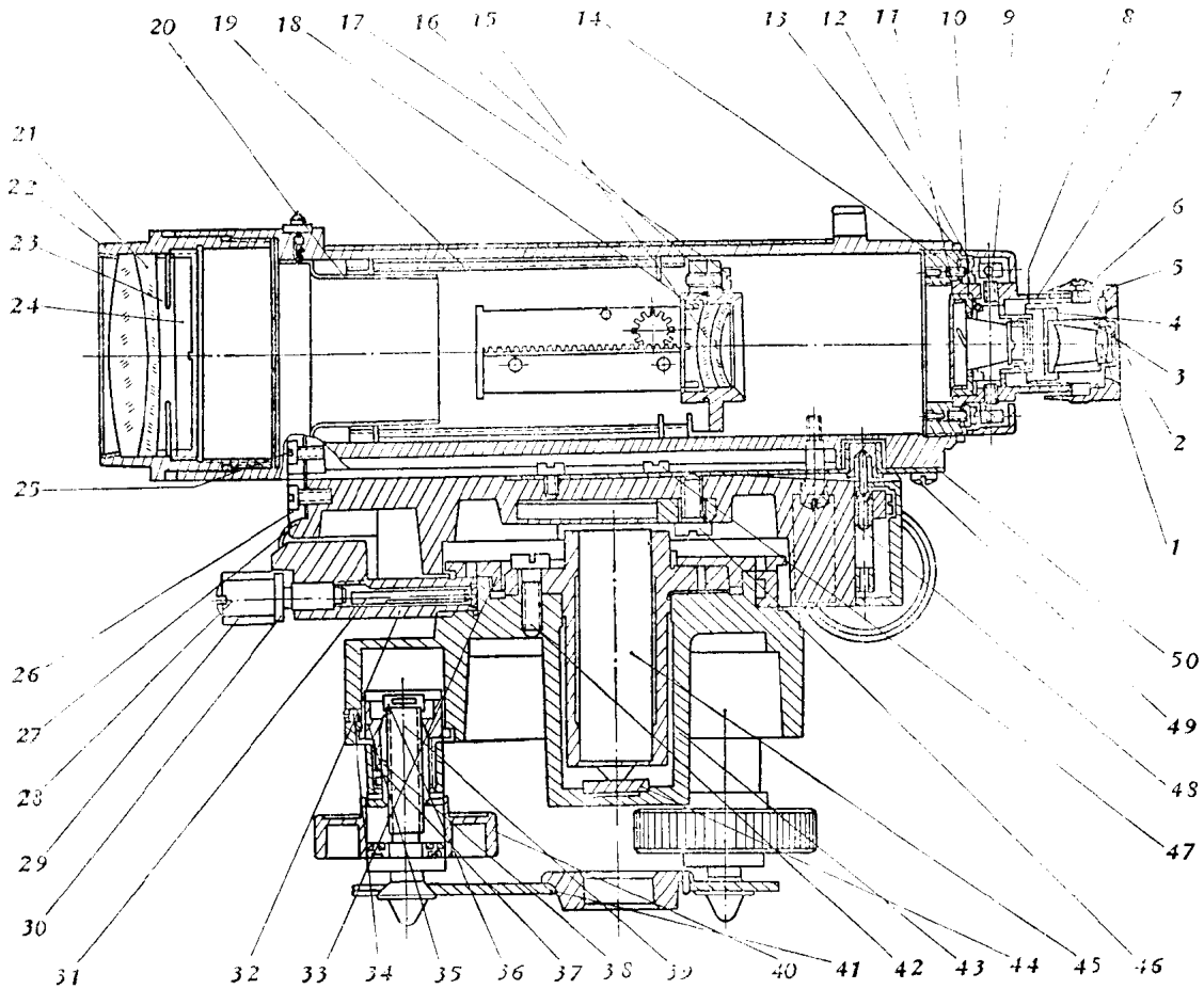
图13-2 CSZ030型水准仪剖面
