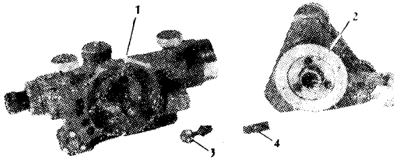
图13-3 竖轴拆卸
