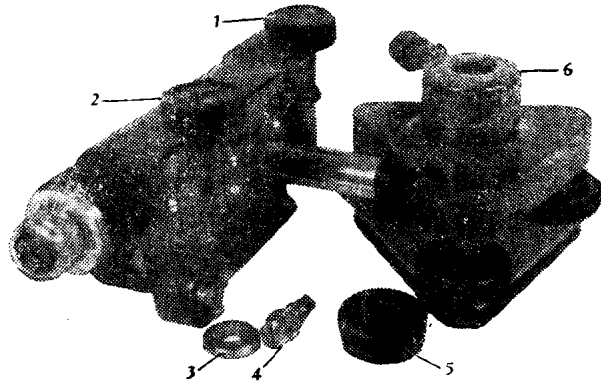
图12-4 竖轴拆卸
