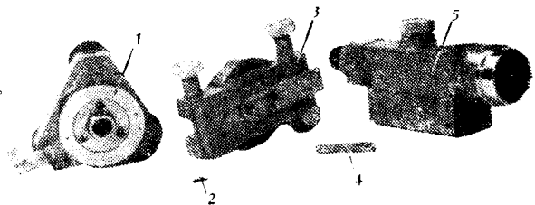
图13-4 基座、托板与望远镜
