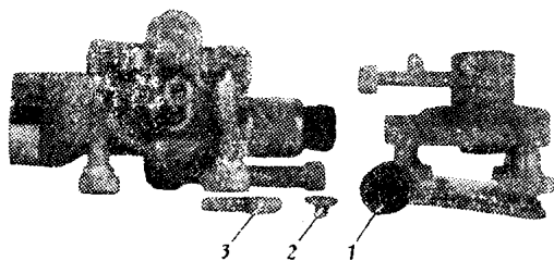
图14-2 竖轴拆卸
