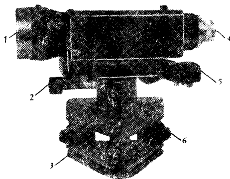
图12-1 水工水准仪外貌
