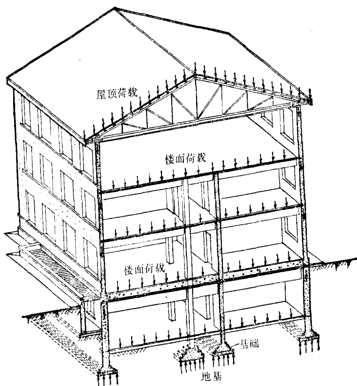
图 1-1 房屋荷载传递示意图
