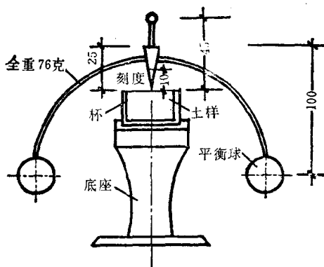
图 2-4 锥式液限仪 (单位: 毫米)
