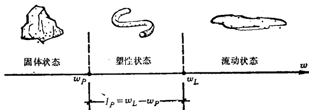
图 2-2 粘性土的状态
