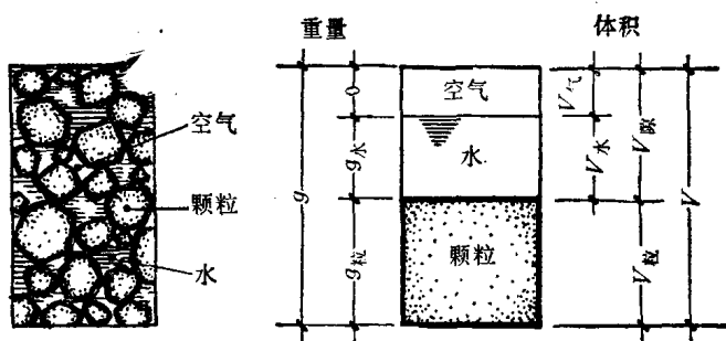
图 2-1 土的三个组成部分示意图
