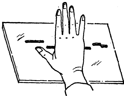
图 2-3 塑限试验
