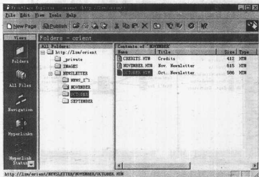
图 1-11 在 Explorer 中拖动文件
