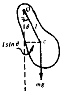
图15-4 复摆
