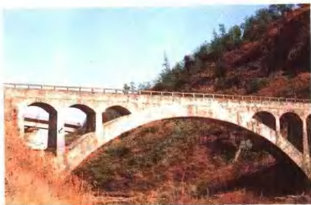
马家河水利配套工程之一 —— 茅塔河渡槽
