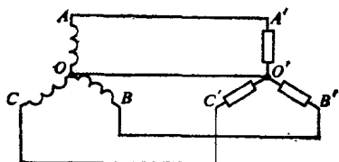
图 1-2 三相交流电的星形接法
