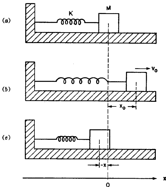
图 1.1 系在弹簧上的质量 M 作水平振动。(a) 弹簧处于松弛状态的平衡位置。(b) 时间 t=0 时的图形, 这时质量 M 被移动了距离 x_0 , 并获得了初速度 v_0 。(c) 经某段时间 t 以后的一般图形。
