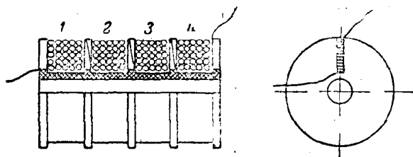
圖 1-1 從操作中分析出裝夾的例子：分段纏繞多層無感線捲。
