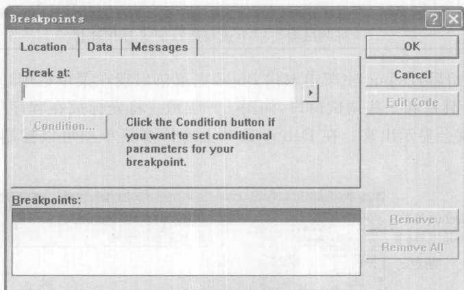
图 1-8 Breakpoints 对话框
