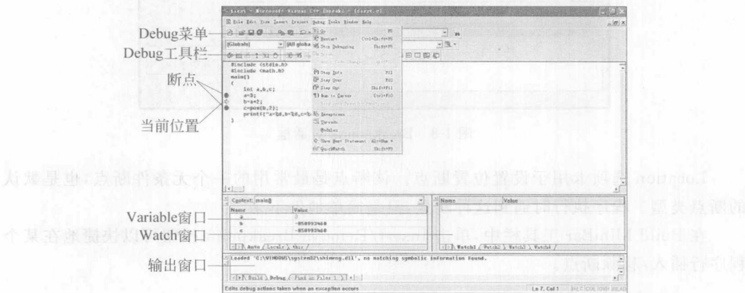
图 1-9 Debug 界面
