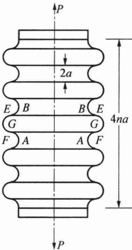
图1 半圆弧波纹管尺寸
