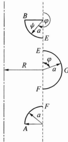
图2 半圆弧波纹管单元坐标
