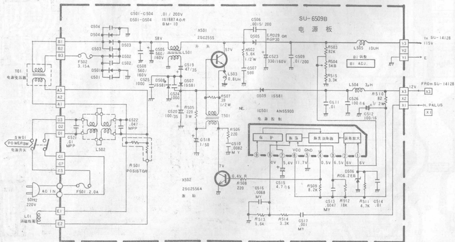
电源单元电路图
