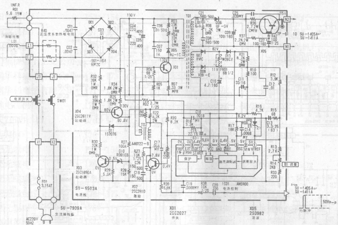
电源单元电路图
