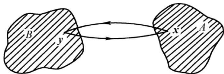
图 1.7 空间 A 一一对应地映射成空间 B 的说明
