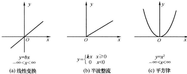
图 1.4 随机变量的函数
