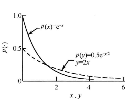
图 1.5 例 1.1 的密度函数
