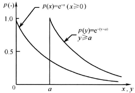
图 1.6 例 1.2 的密度函数
