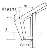
(K) 木扶手与立柱连接示意图
