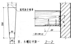
侧立面图
