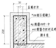
⑫ 踏步边缘现制踢脚线作法
