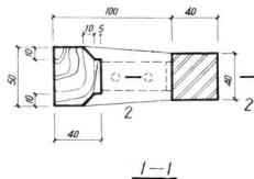
木扶手样图
