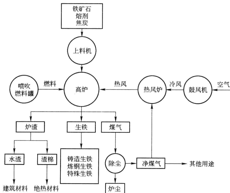
图 1-1 高炉炼铁生产工艺流程
