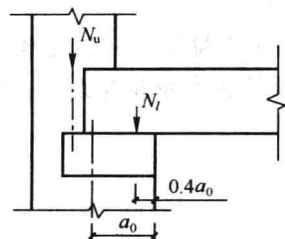
图 4.2.5 梁端支承压力位置
