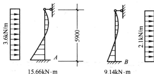
图 6.1.5 l=18\text{m} 车间柱底弯矩
