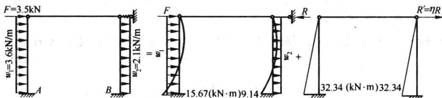
图 6.1.7 l=36\text{m} 车间排架计算简图及柱底弯矩
