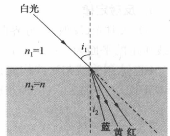
图 1.3 光在折射时出现色散现象
