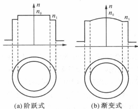
图 1.8 光纤折射率的不同分布
