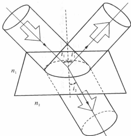
图 1.1 光的反射和折射
