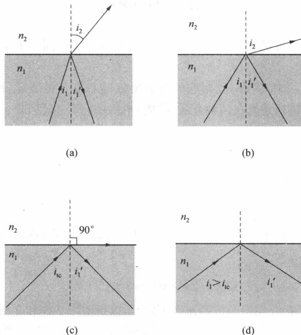
图 1.5 n_2 < n_1 , 光从光密介质射入光疏介质时的四种情况
