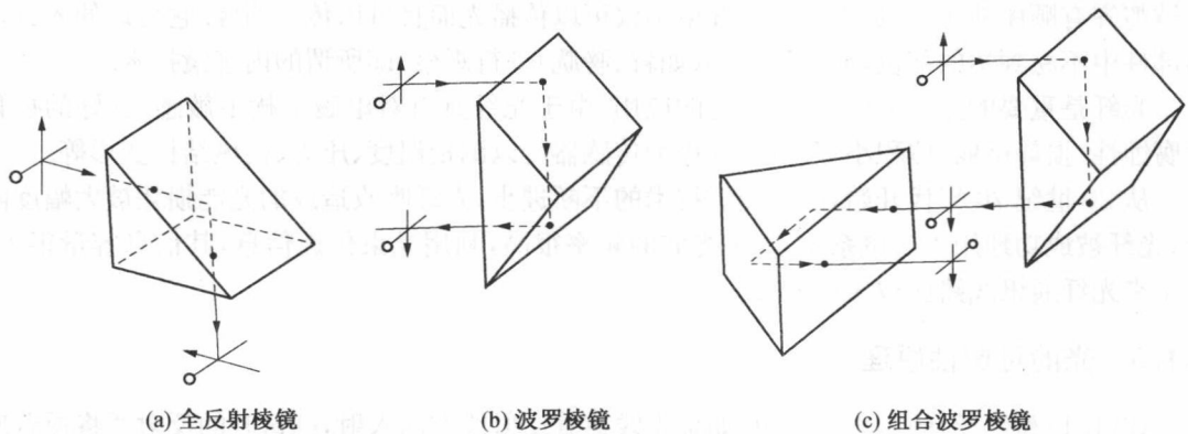
图 1.6 三种反射棱镜
