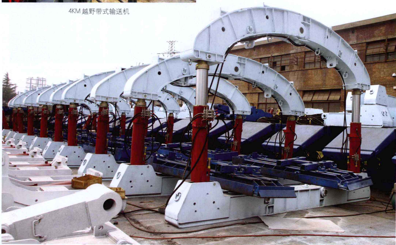
防冲液压支架
