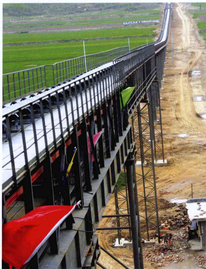
4KM 越野带式输送机
