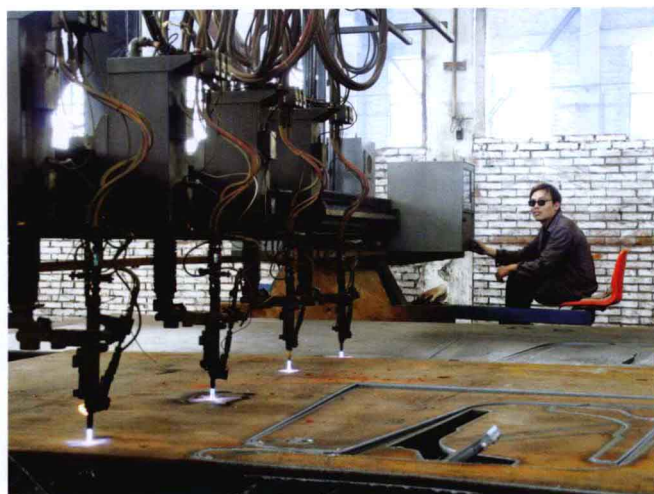
员工操作数控火焰切割机
