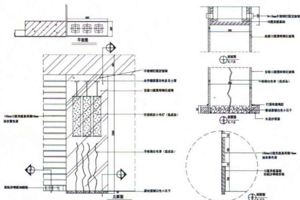
●餐厅屏风隔断立面图
