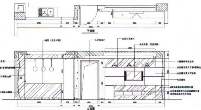
●客厅电视墙立面图
