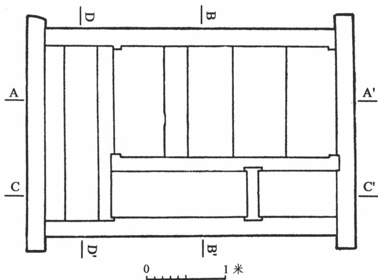
圖四 M168 棺槨結構平面圖
