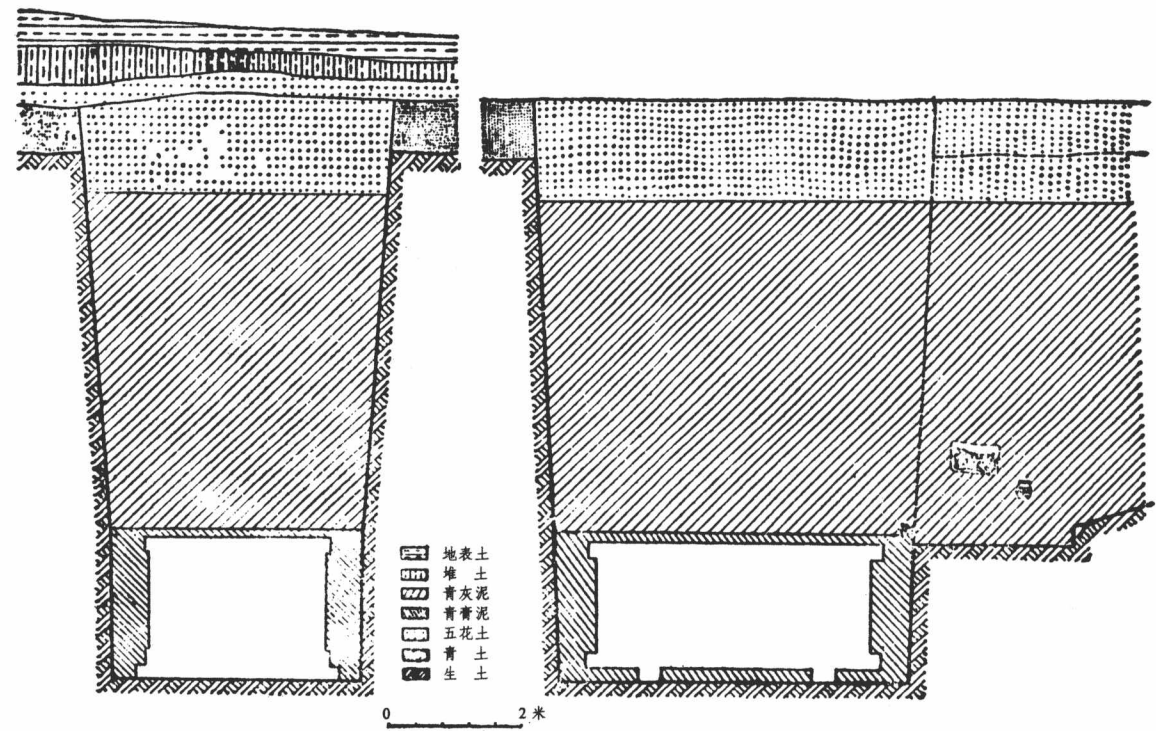
圖三 M168 橫剖面圖(左)與縱剖面圖(右)
