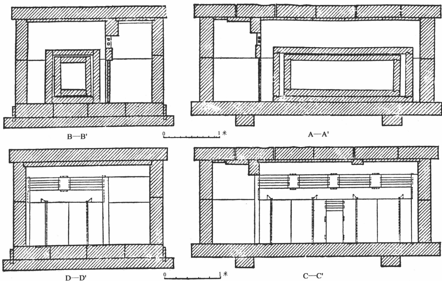
圖五 M168 棺槨結構圖
