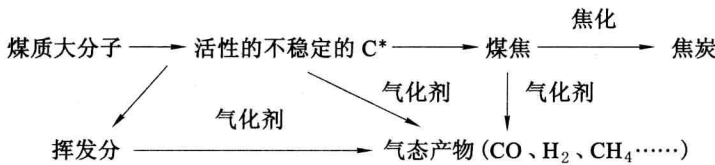
图 1-1 煤质分子的变化
