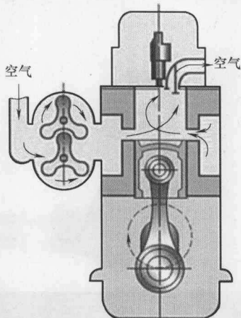
(2) 增压式发动机
