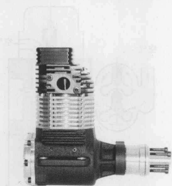
(1) 单缸发动机
