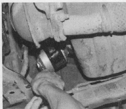
(5) 更换机油滤清器
