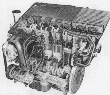
(2) 多缸发动机
