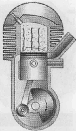
(1) 自然吸气发动机
