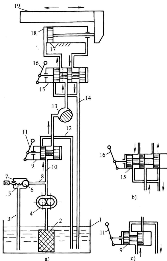
图1-2 磨床工作台液压系统的工作原理
