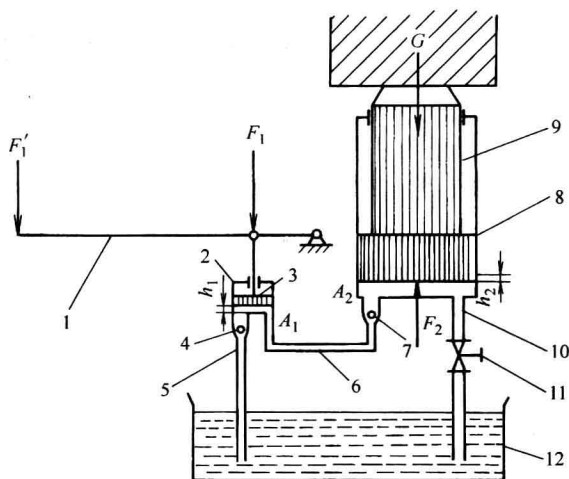
图 1-1 液压千斤顶的工作原理
