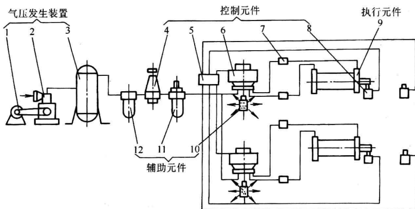
图 1-3 典型气动系统的组成
