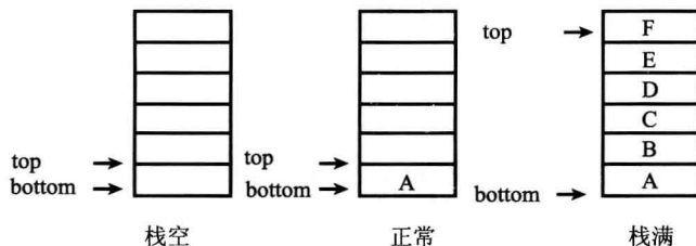
图 0-1 栈的状态
