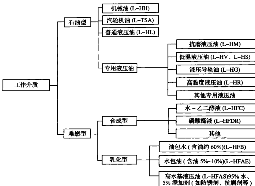
图 2-1 工作介质的种类
