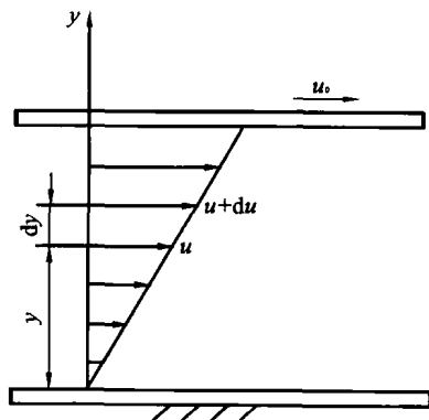
图 2-2 液体黏性示意图
