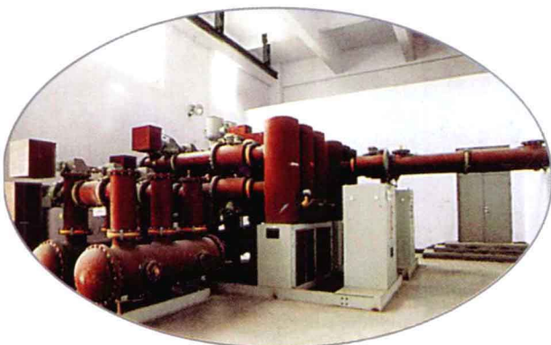
济钢 110Kv 变电站采用国内领先的 GIS 组合电器
