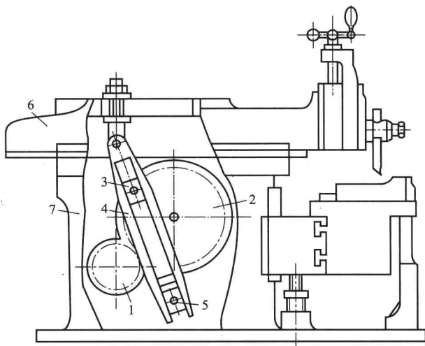
图1-1 牛头刨床
