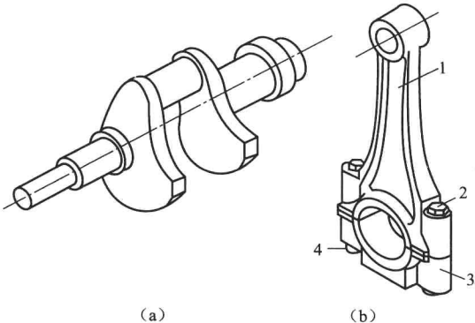
图 1-3 零件和构件
