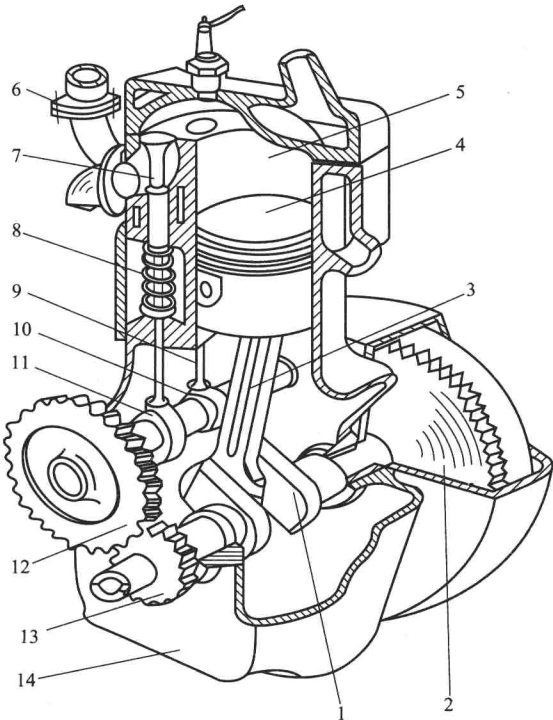
图 1-2 单缸内燃机
