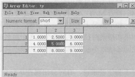
图 1.8 数组编辑器
