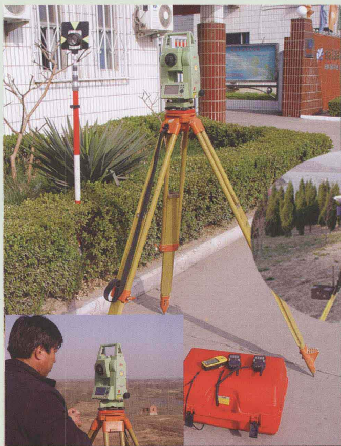
先进的测量设备—GPS、全站仪
