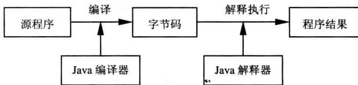
图 1.1 Java 程序的上机步骤
