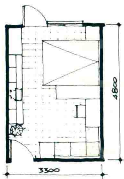
设计后平面图
