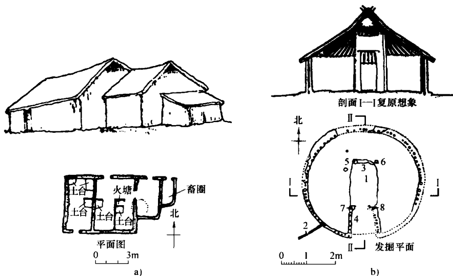
图 1-4 大河村、半坡遗址房屋的想象复原外观
