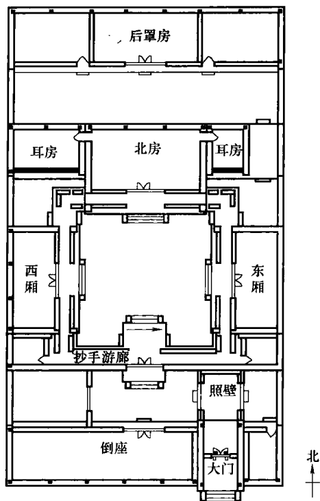
图 1-6 明、清时期北京典型四合院平面图
