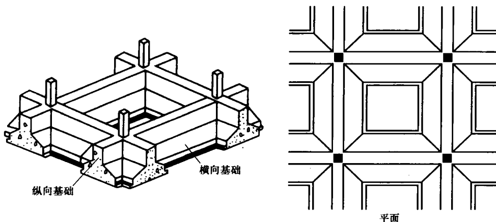
图 1-9 柱下条形基础
