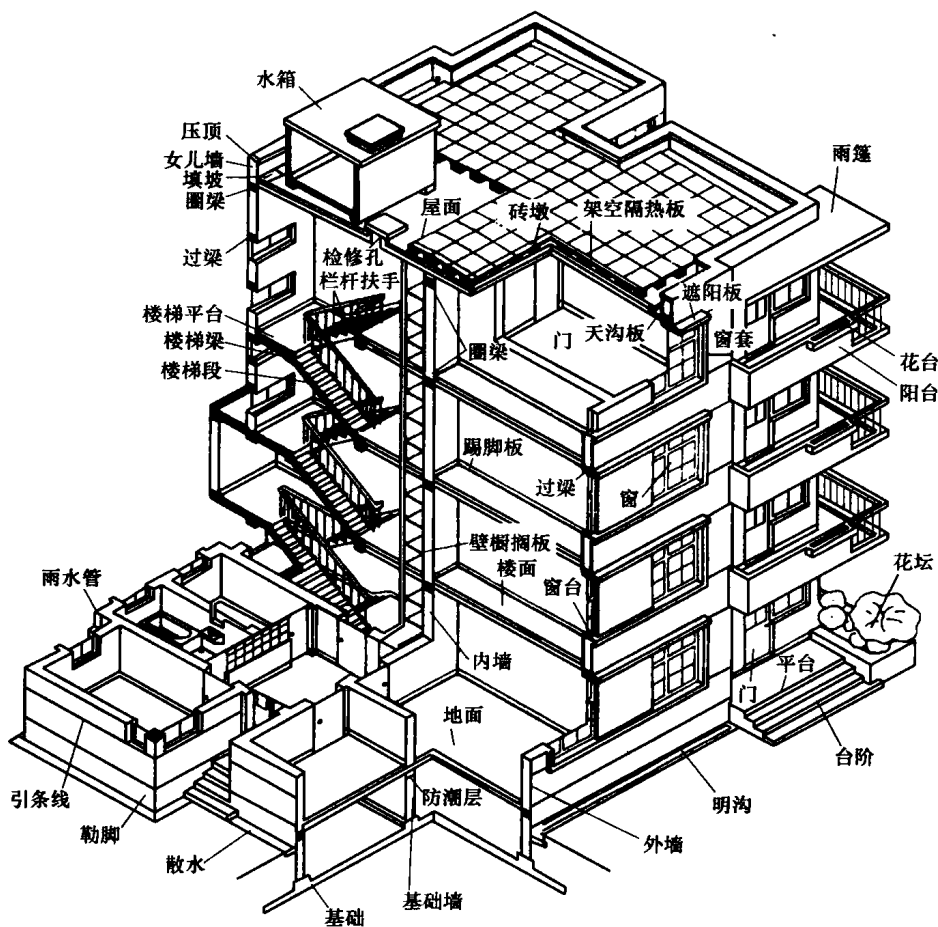
图 1-7 房屋构造示意图
