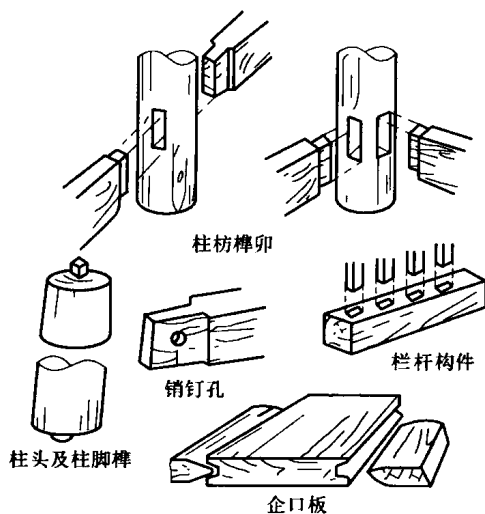
图 1-3 河姆渡遗址榫卯技术
