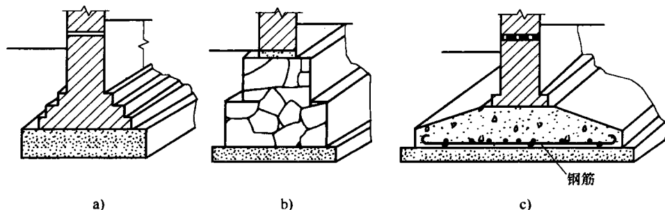
图 1-8 墙下条形基础
