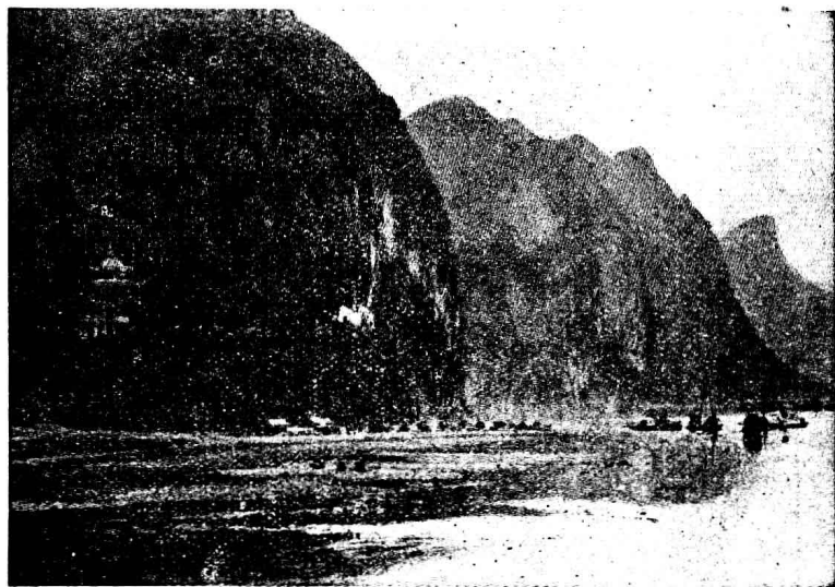
圖四、 廣西桂林石灰山 ，除圖中之渾圓者外，亦有極峻削的峯巒，河谷中多石灘。
