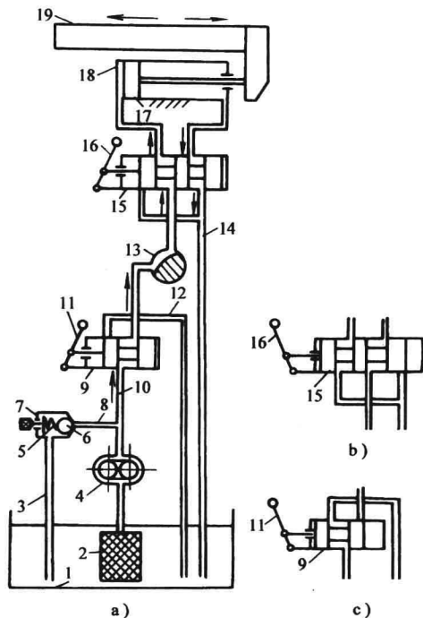
图 0-2 机床工作台液压系统的工作原理图
