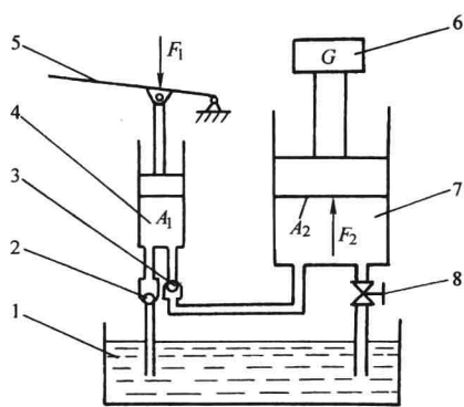
图 0-1 液压千斤顶示意图
