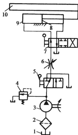
图0-3 机床工作台液压系统的图形符号图
