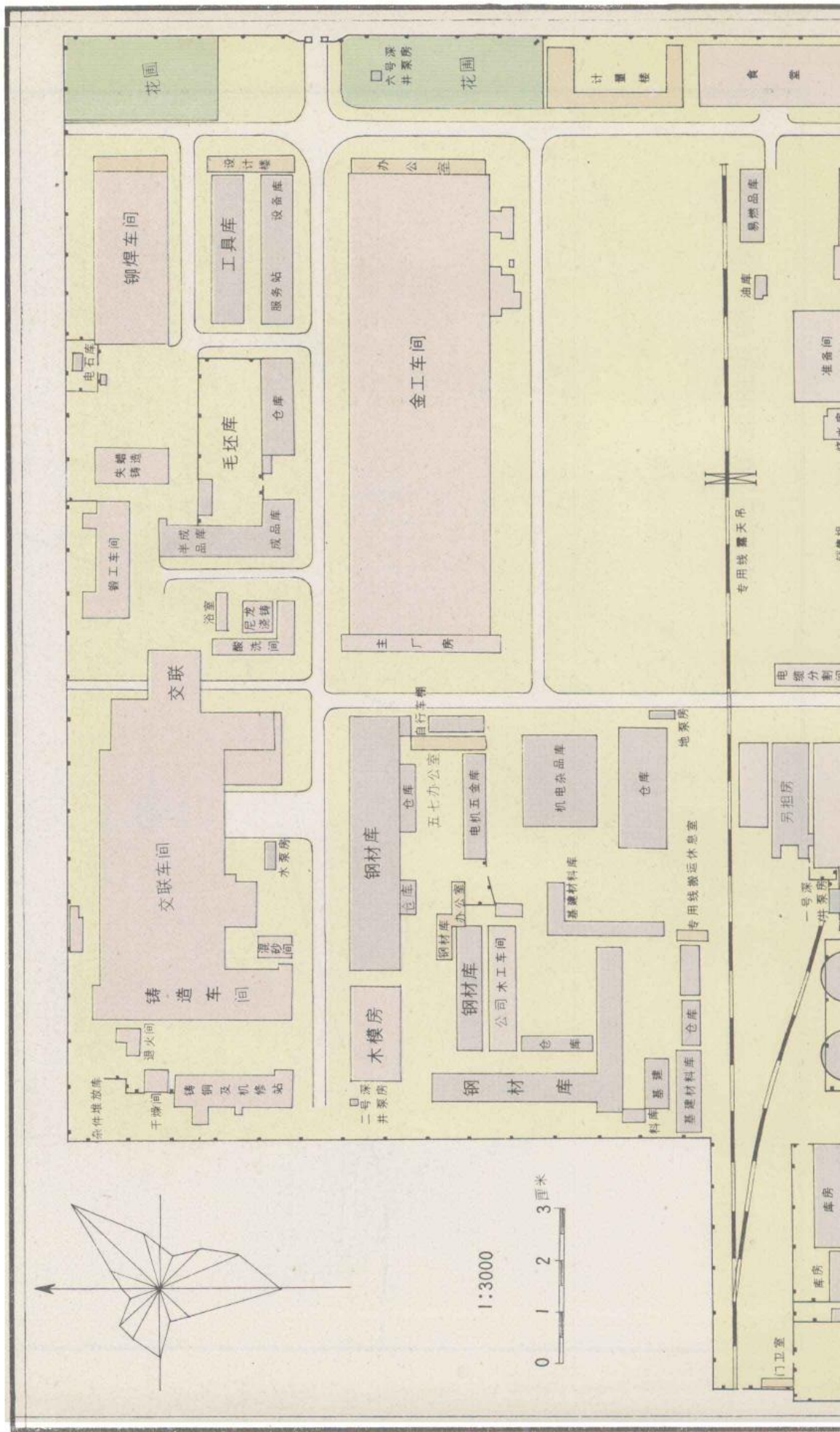
电缆厂厂区总平面图
