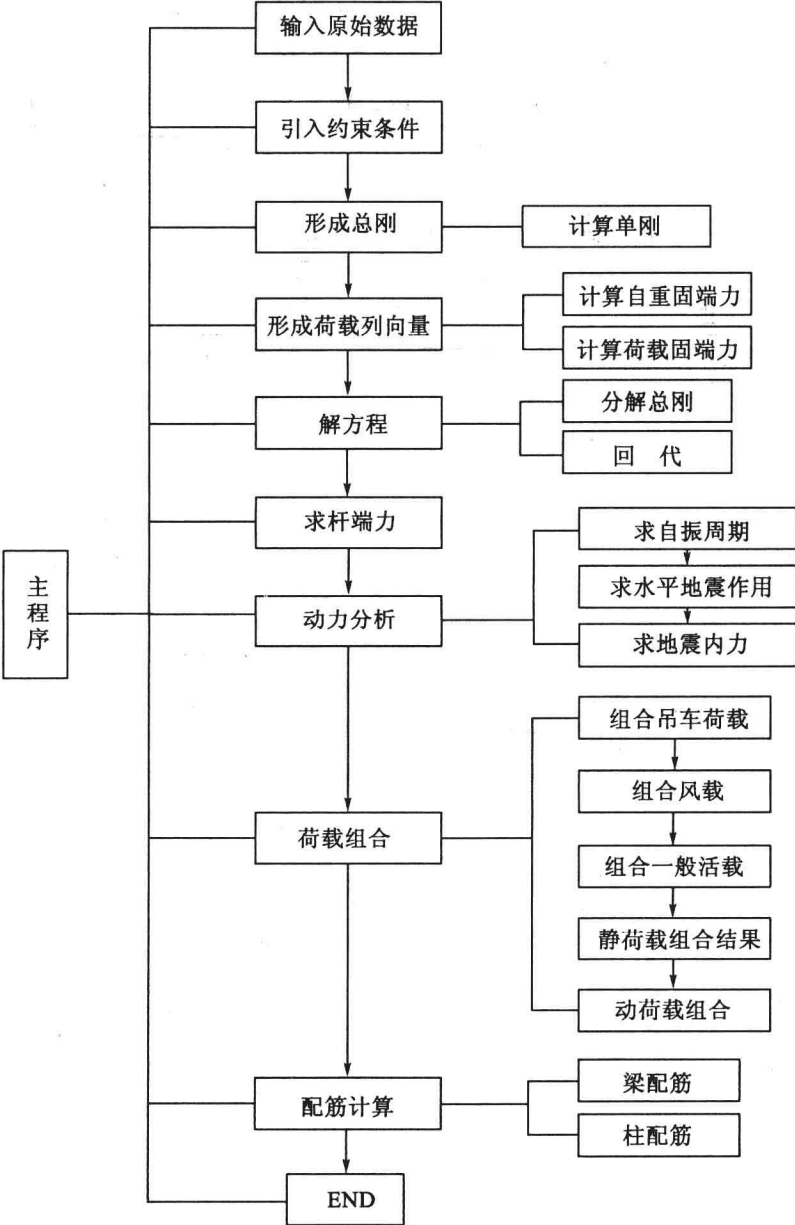
图 1-1 框架结构分析程序总框图
