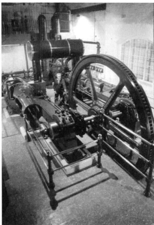
图1.1.1 18世纪的蒸汽轮机 位于伦敦克佑桥(Kew bridge) 蒸汽博物馆的实物照片
