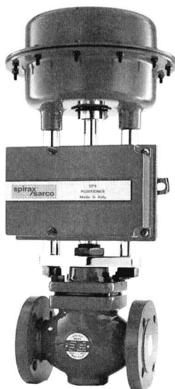
图1.1.4 典型的带定位器的的气动二通控制阀
