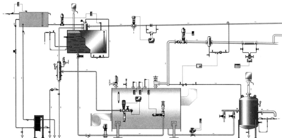
图1.1.5 现代蒸汽锅炉房
