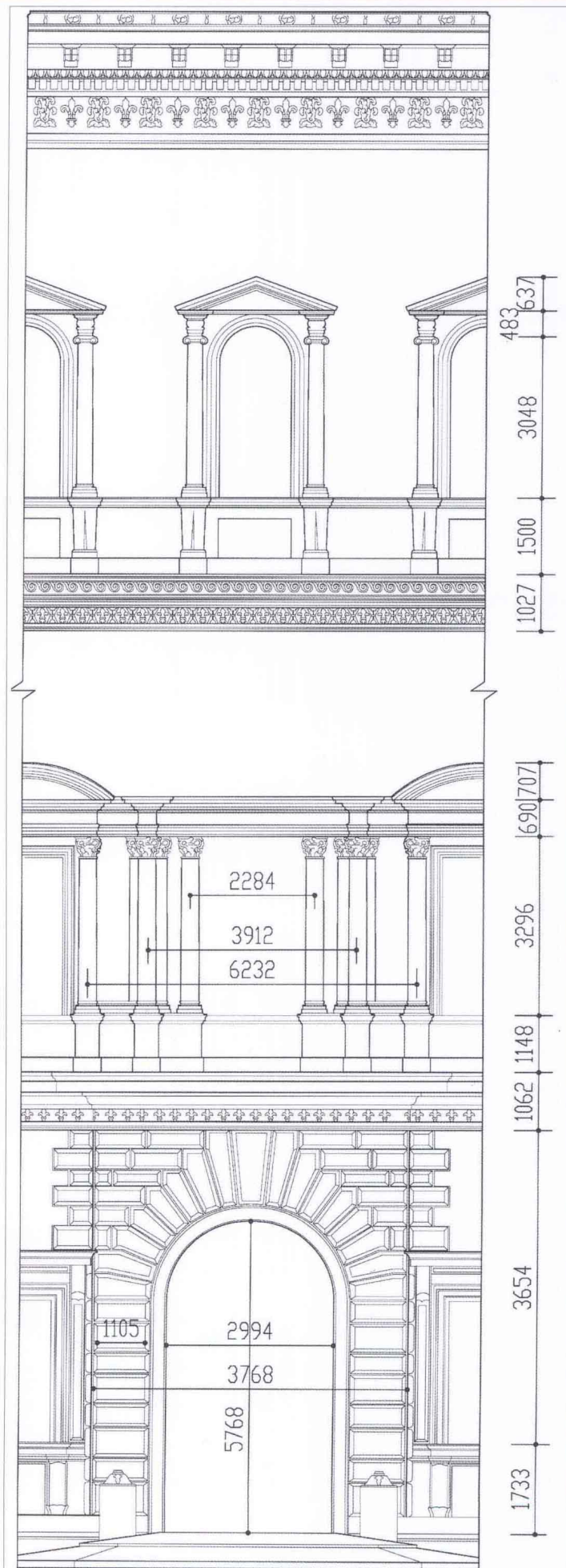
正面中间立面
