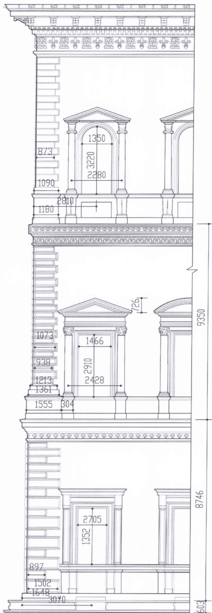
正面拐角处立面
