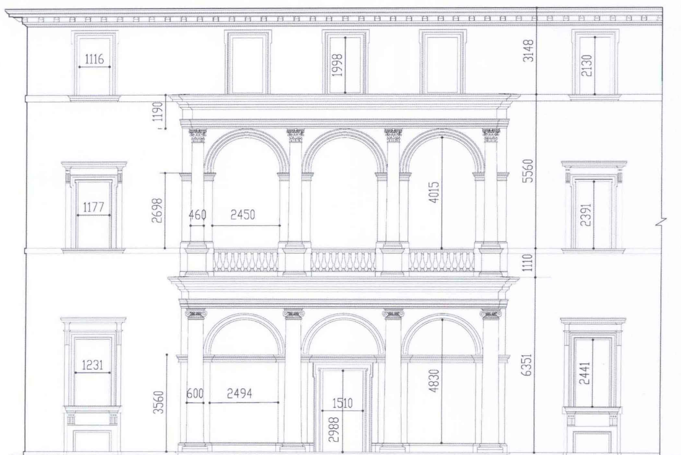
靠近花园的墙体正立面
