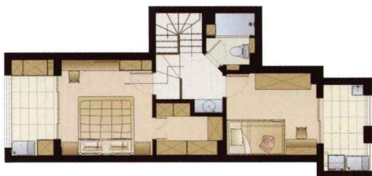
二层平面图
