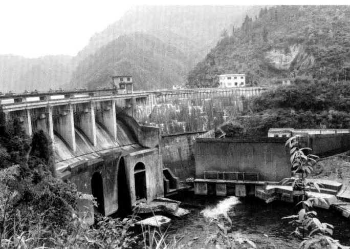
图22 1993年7月，角口水电站竣工投产
