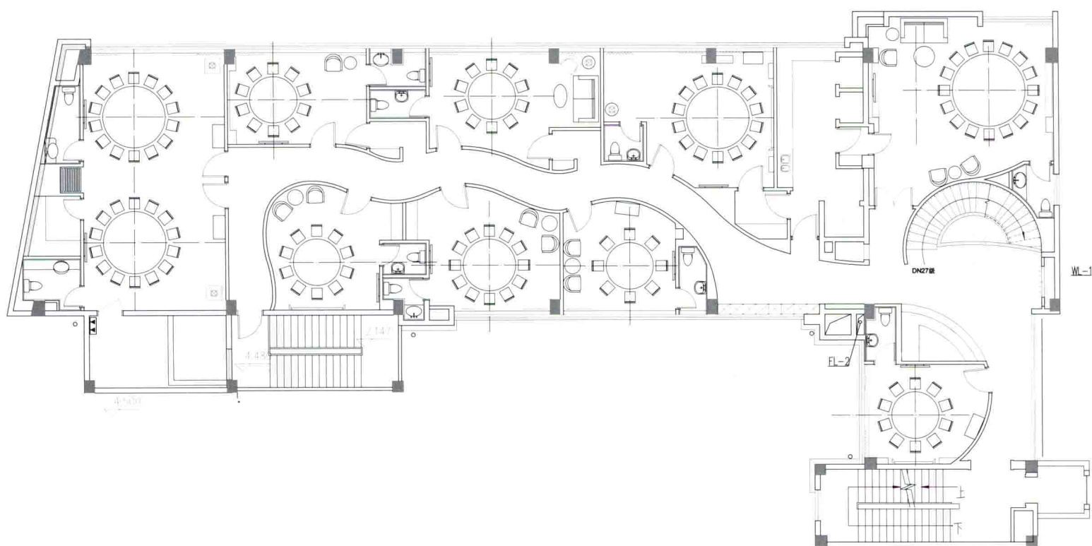
平面图
