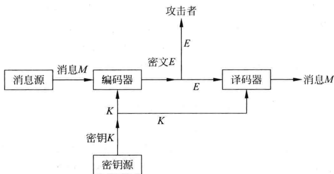
图2 Shannon的通用保密系统方案
