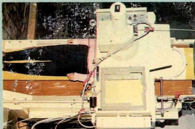
F99—IA500MA 带电视 X 线机
