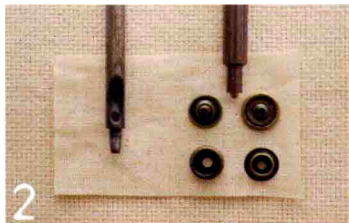
2 两两一组，使用尺寸相对应的四合扣工具敲打定型。
